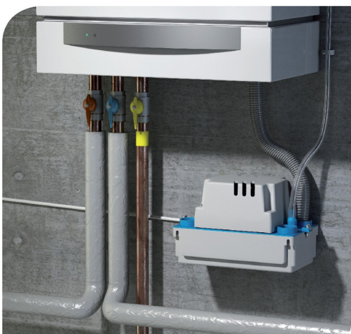
Refolements vertical et horizontal : ↑ 4,5 m → 50 m
