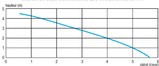
Courbe de débit Sanicondens Eco et Sanicondens Pro
