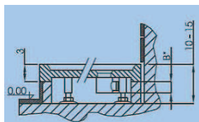
Posé sur pieds réglables avec habillage carrelé
