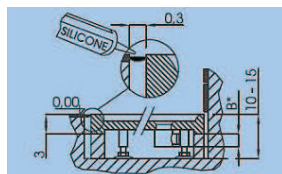
Encastré et posé sur pieds réglables
