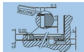
Encastré et posé sans pieds réglables
